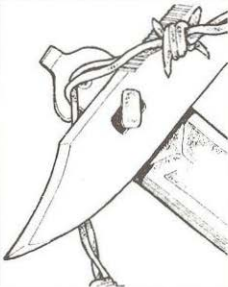
Bayonett KCB 77 "L" M 1, lange Ausführung mit Schere Bayonet KCB 77 "L" M 1, long execution with scissors Baïonnette KCB 77 - L - M 1, longue, avec ciseaux
